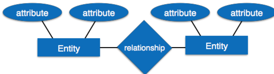
Fig 8: ER Model
